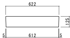
J I S側溝500用蓋
