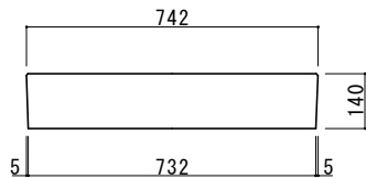
深溝側溝600用蓋
