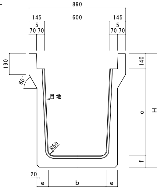
正面図
