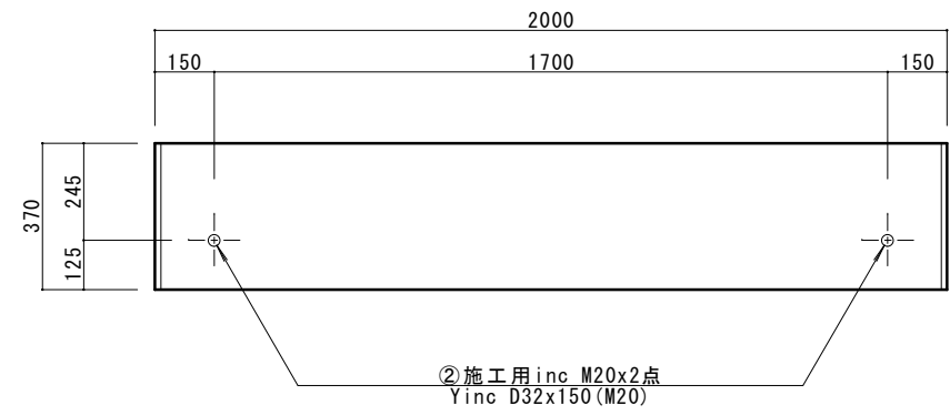
正面図
