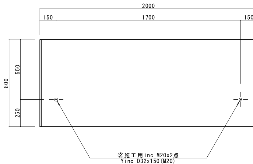
正面図
