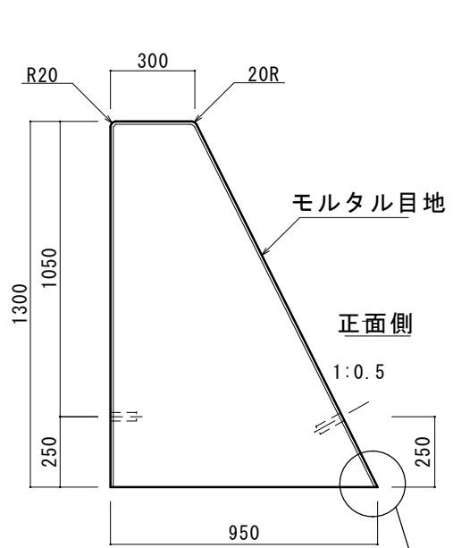
目地形状
