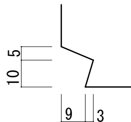
目地形状
