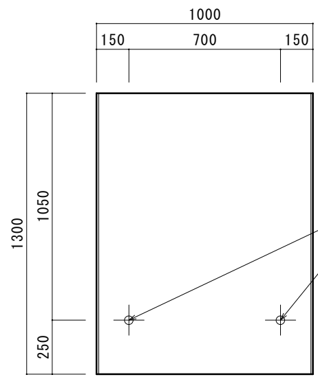
背面図
