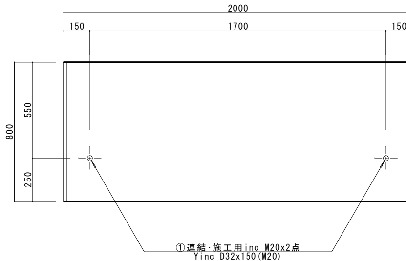
正面図
