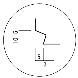
目地形状
