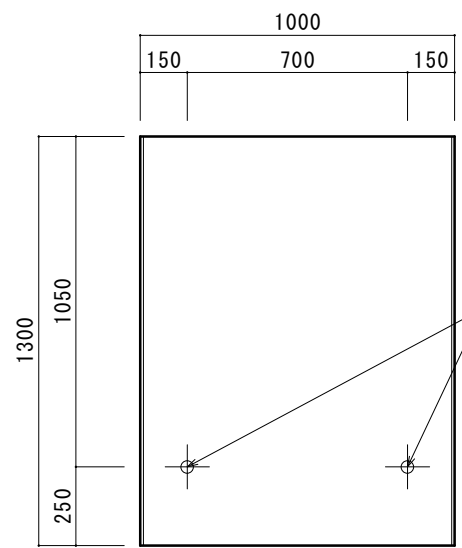
正面図
