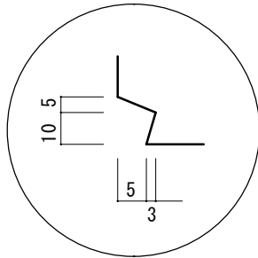
目地形状
