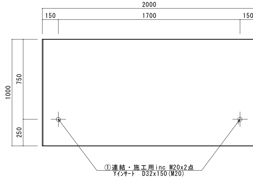
背面図
