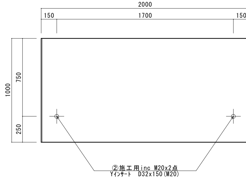
正面図
