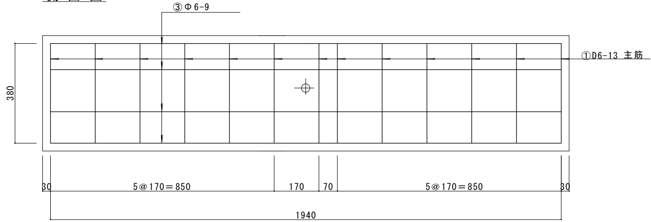
側面図
