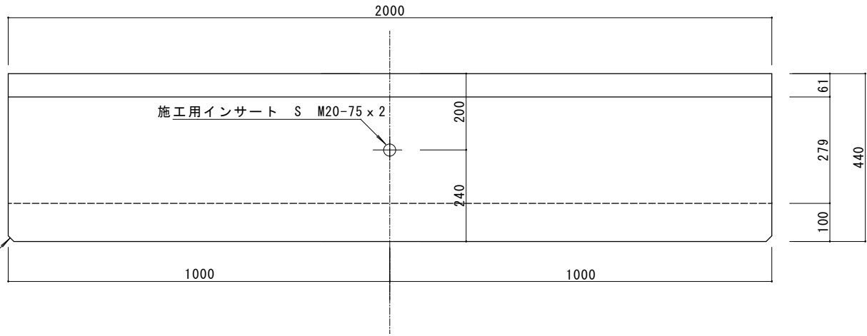
側面図
