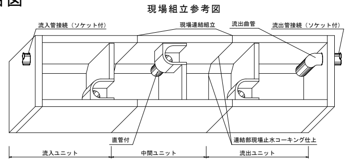
ユニット連結部詳細図
