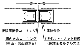
連結金物詳細図
