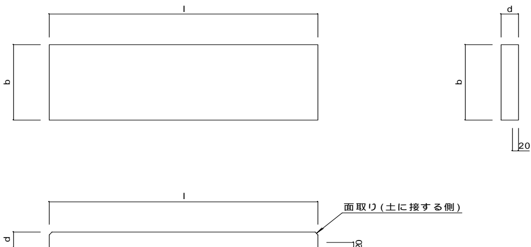
土留柵板 寸法一覧表
