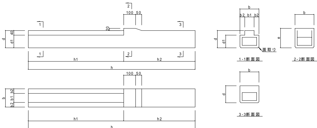
土留柵杭 寸法一覧表
