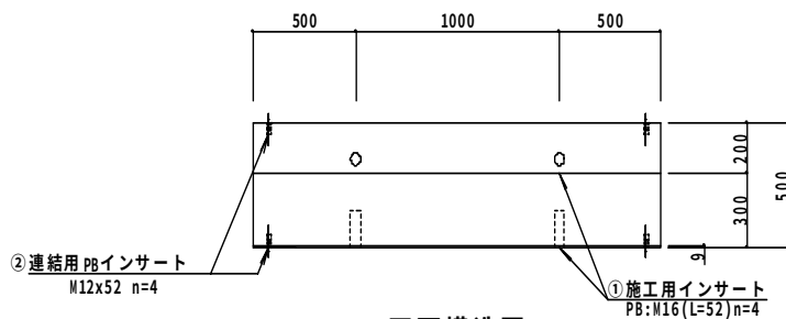
正面構造図
