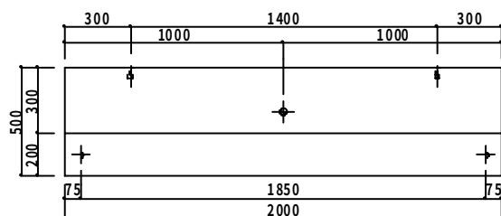
正面図
