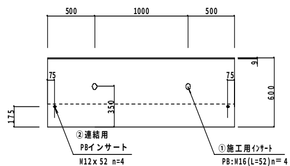
正面構造図
