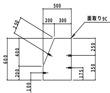
側面構造図
