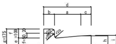
コンクリートL型，鉄筋コンクリートL型 寸法一覧表
