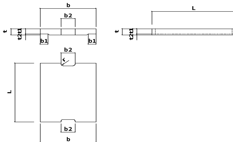
U型側溝蓋 寸法一覽表
