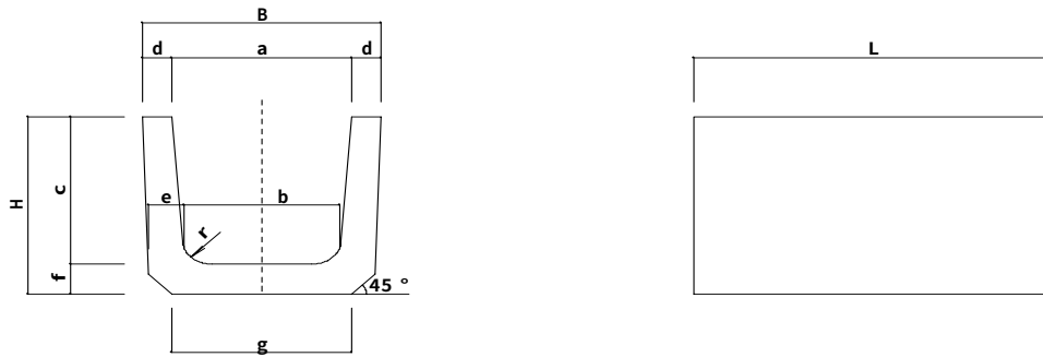
U型側溝 寸法一覽表
