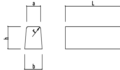
両面歩車道境界ブロック
