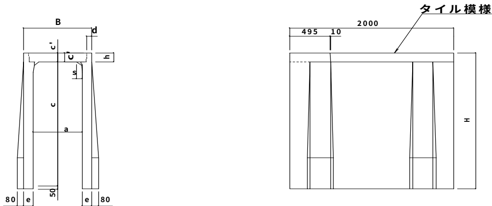
アートVS側溝 600x1600～2000 寸法一覧表
