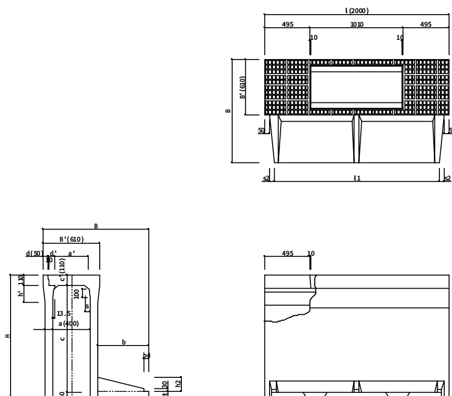
土留付大型VS 寸法一覧表
