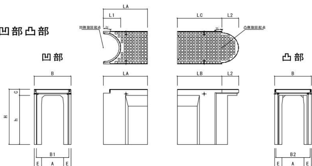
フレキシブル側溝 寸法一覧表
