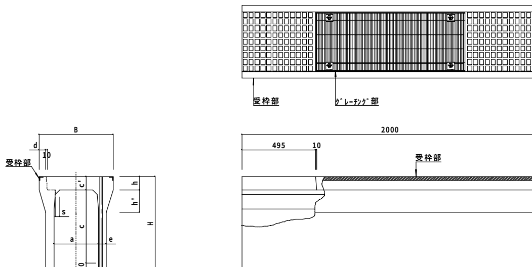
横断AVS側溝 寸法一覧表
