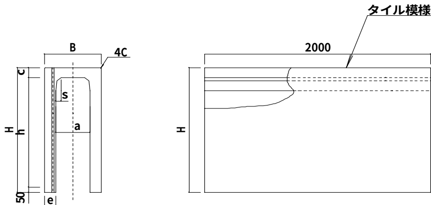
暗渠型VS 寸法一覧表
