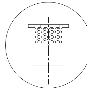
排水金具詳細図
