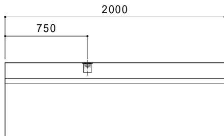
側面図 S=1/35
