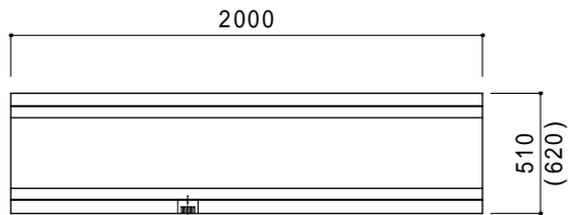
平面図 S=1/35
