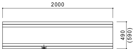
平面図 S=1/35
