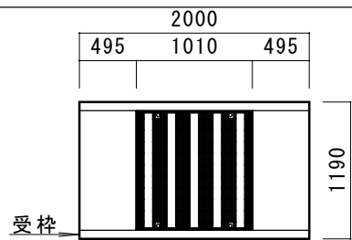
平面図 普通目 S=1:60
