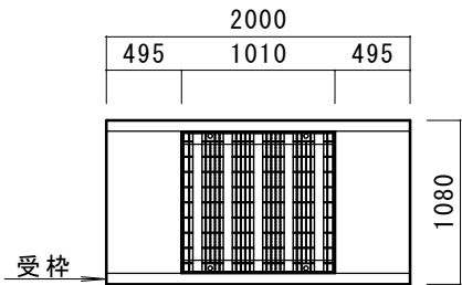
平面図 普通目 S=1:55
