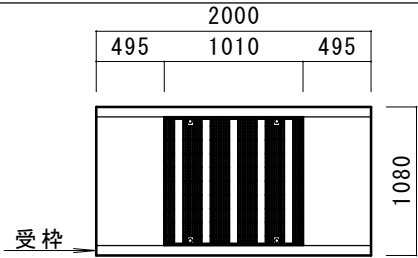
平面図 細目 S=1:55
