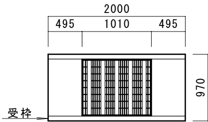
平面図 普通目 S=1:55
