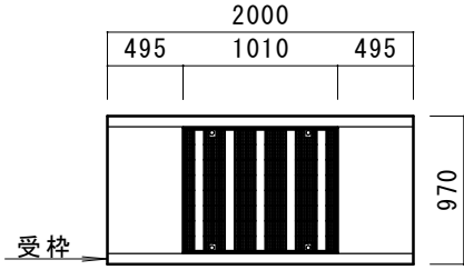
平面図 細目 S=1:55
