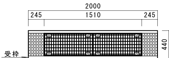
平面図 普通目 S=1/35
