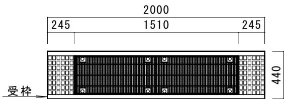
平面図 細目 S=1/35
