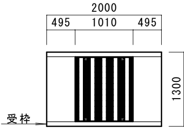
平面図 普通目 S=1:65
